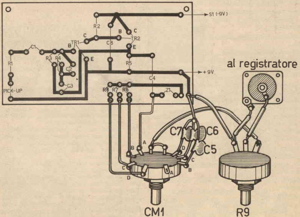
Fig. 2 - Schema pratico
